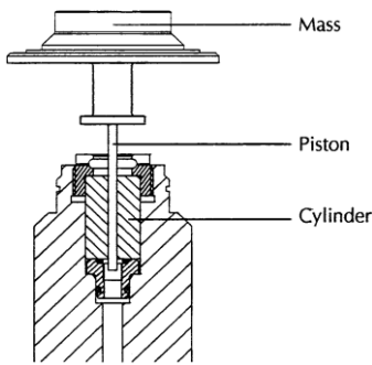
图 1. 活塞压力计原理图
